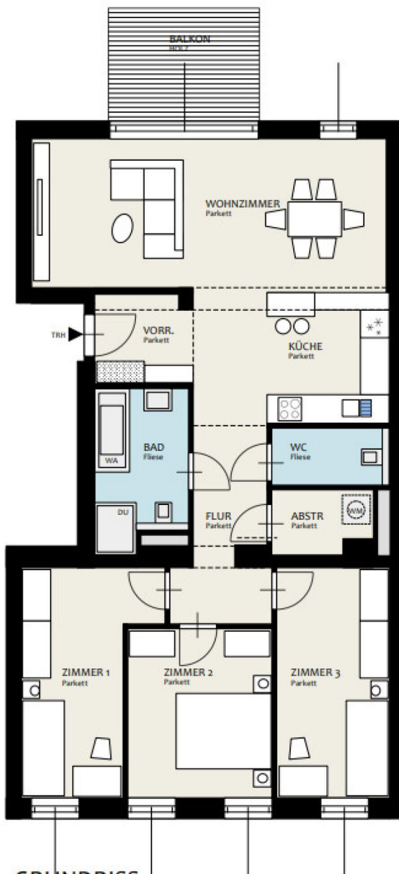
GRUNDRISS 3. OBERGESCHOSS
